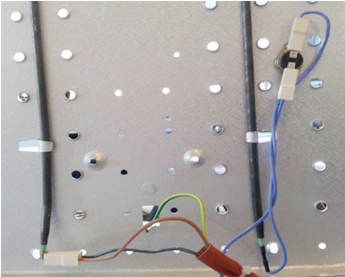
Connexion résistance et thermostat du plateau
